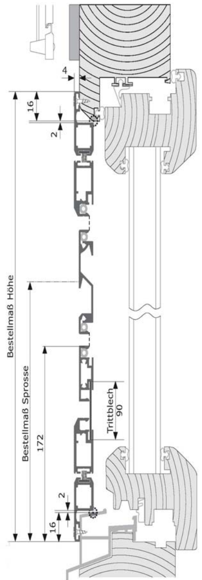
Profil 4040
