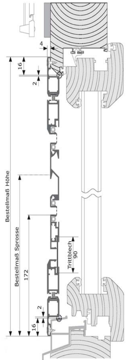
Profil 4040
