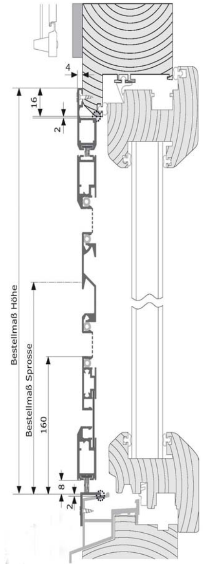
Profil 4040
